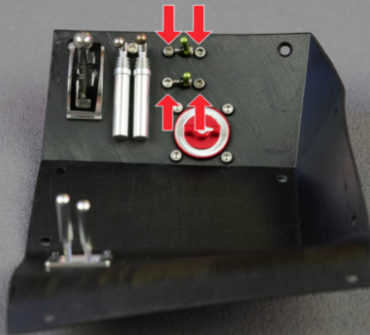
杯頭內六角M1.6*4 4顆
